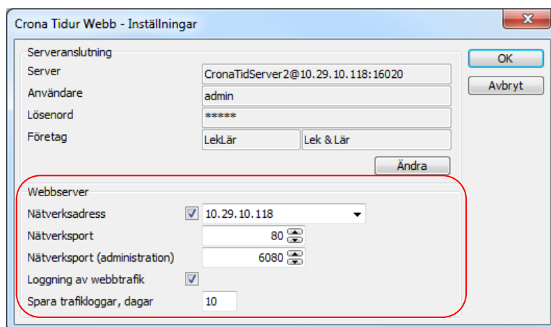
Dialogrutan för inställningar av webbservern.
